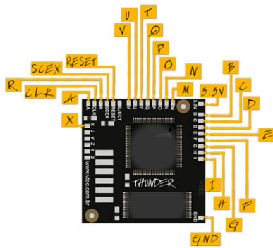
THUNDER chip pinout Os pontos acima devem ser conectados a seus respectivos no diagrama
