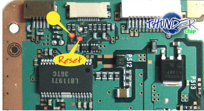
THUNDER chip pinout Os pontos acima devem ser conectados a seus respectivos no diagrama
